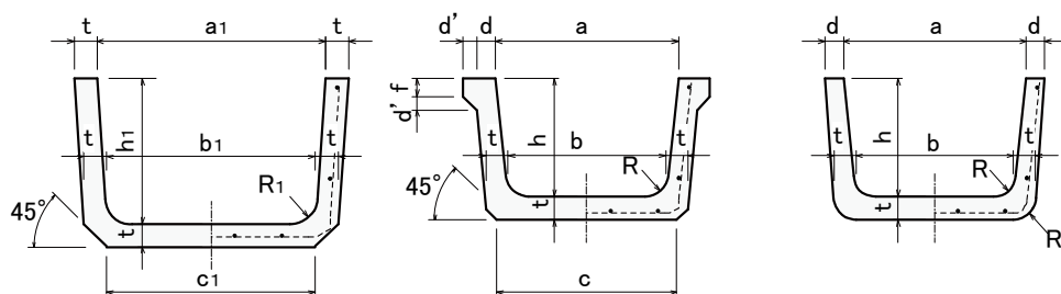
ソケット部断面
