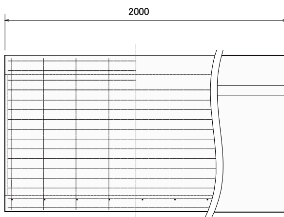
目地詳細
